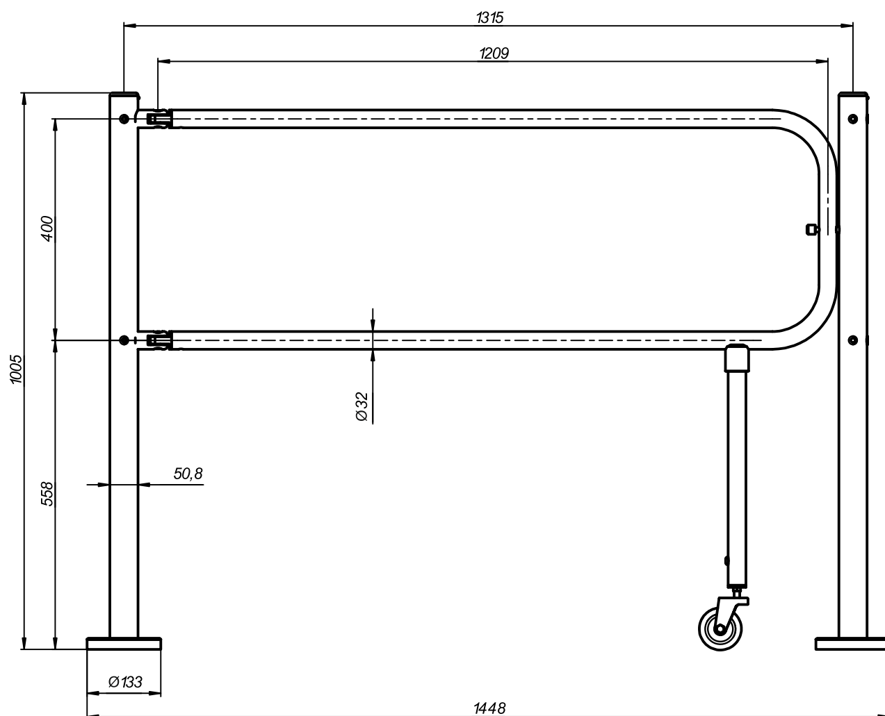
Рисунок 1. Габаритные размеры секции «Антипаника ХТА-01».
