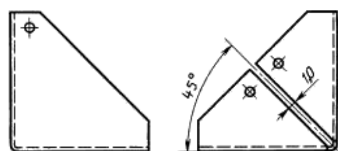
Угольник правый
