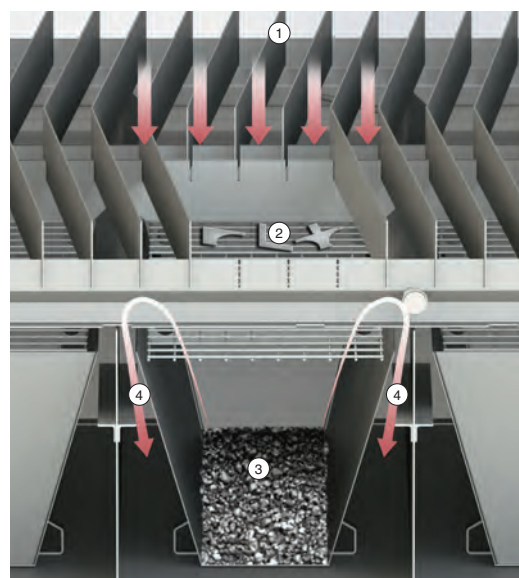
Поперечный разрез модуля MBC
