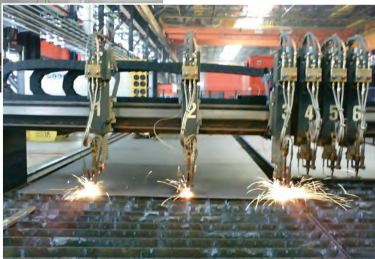
Пример внедрения двухрядного стола в комплекте с фильтром MDB
