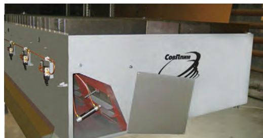
Модуль MBC со снятой заглушкой воздушного канала и без кожуха пневмораспределителей
