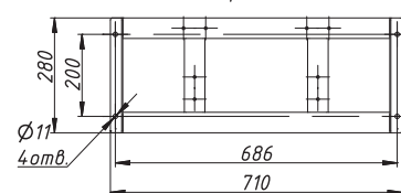
Размеры подставки
