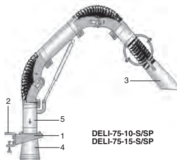
Исполнение S (над опорой)
