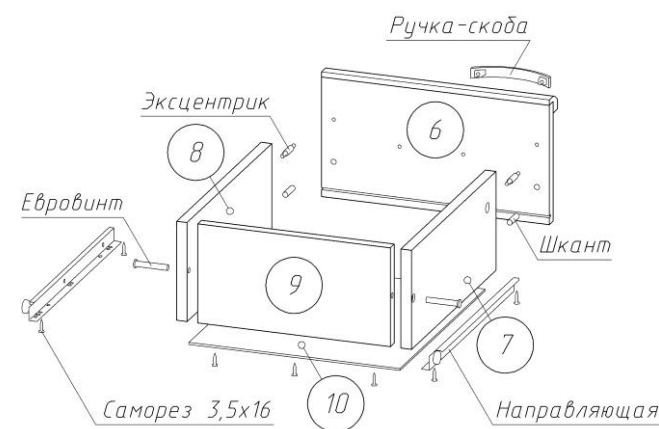
Рисунок 2 – Сборка ящика
