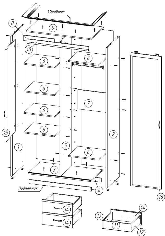
Рисунок 1 – Сборка каркаса
