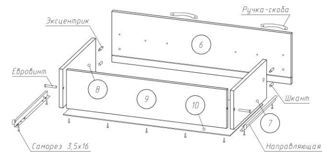
Рисунок 2 – Сборка ящика
