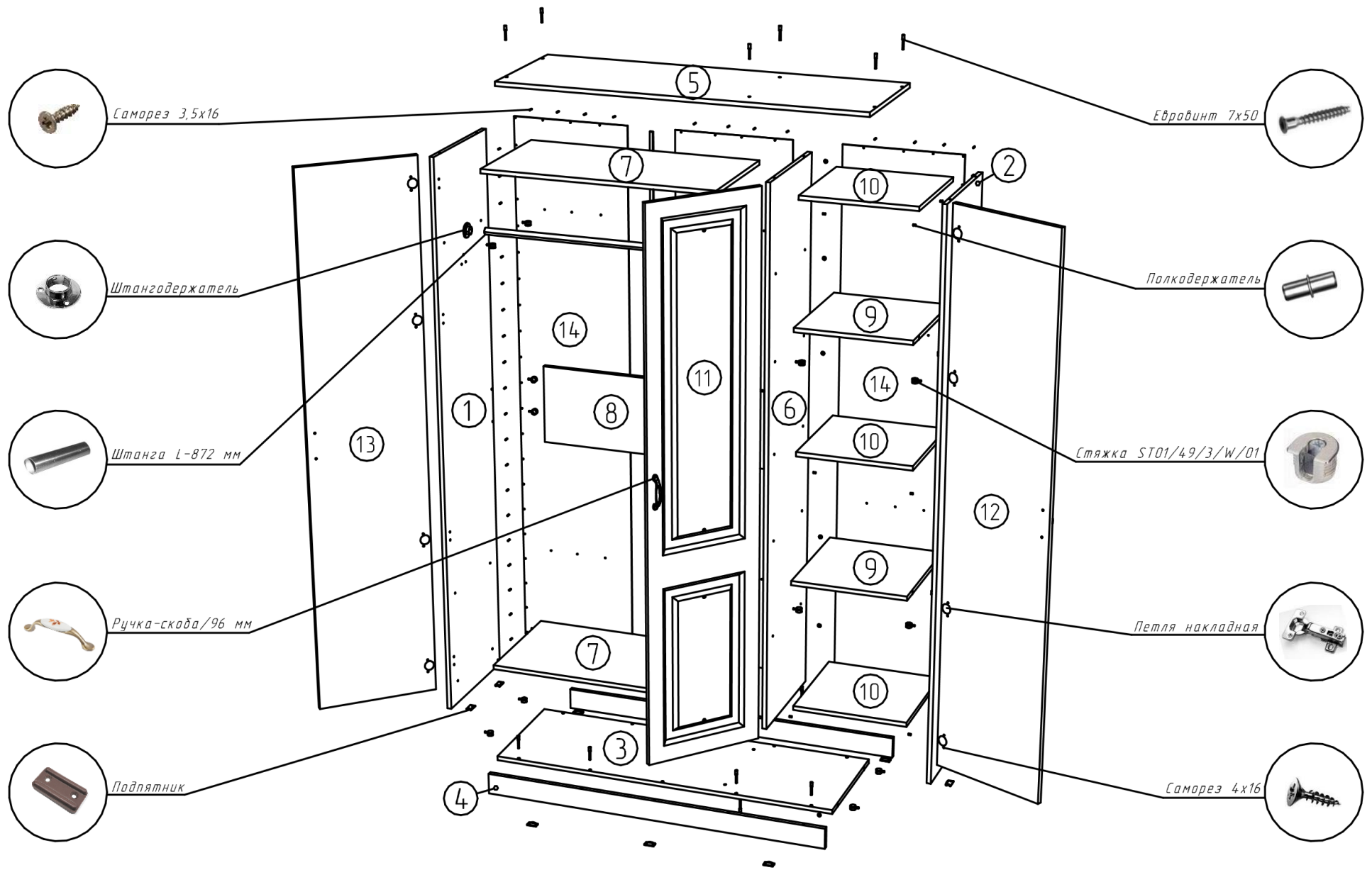
Рисунок 1 – Сборка каркаса
