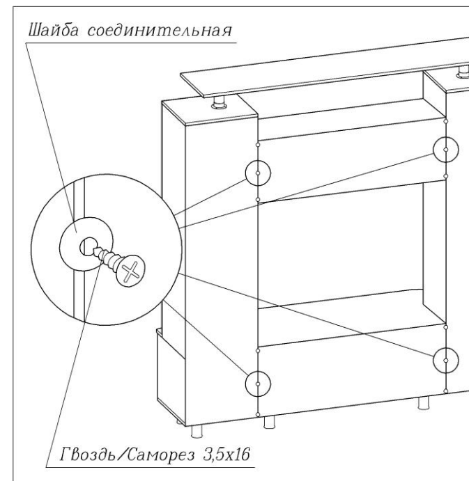
Рисунок 2 – Монтаж ДВП
