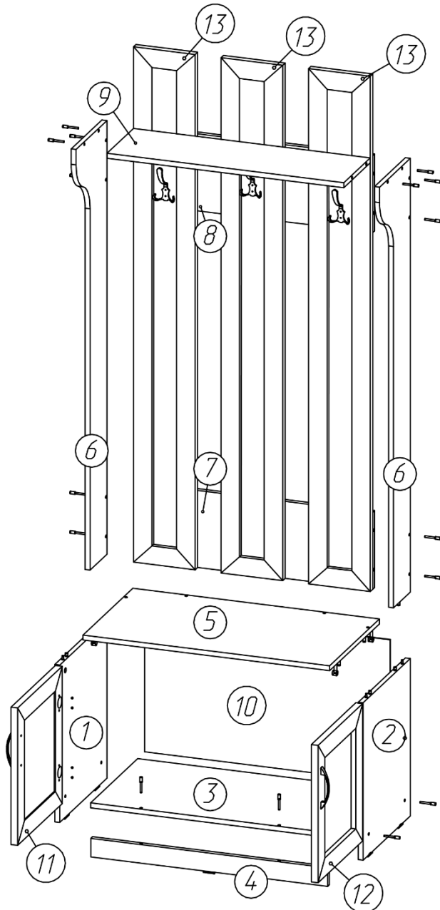
Рисунок 1 – Сборка каркаса
