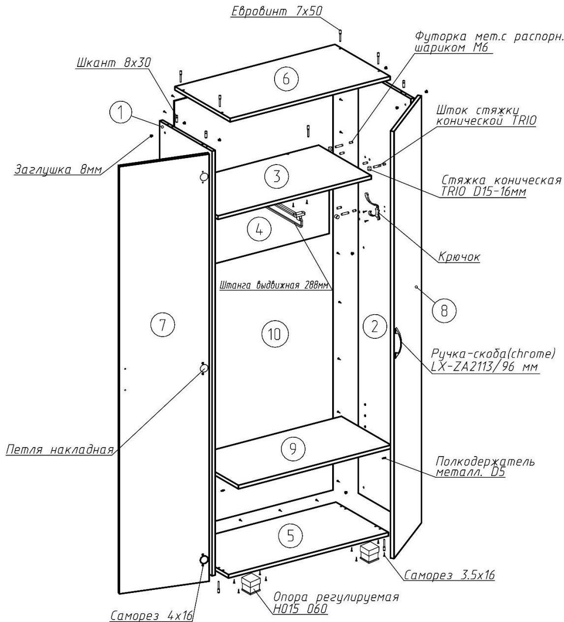
Рисунок 1 – Сборка каркаса
