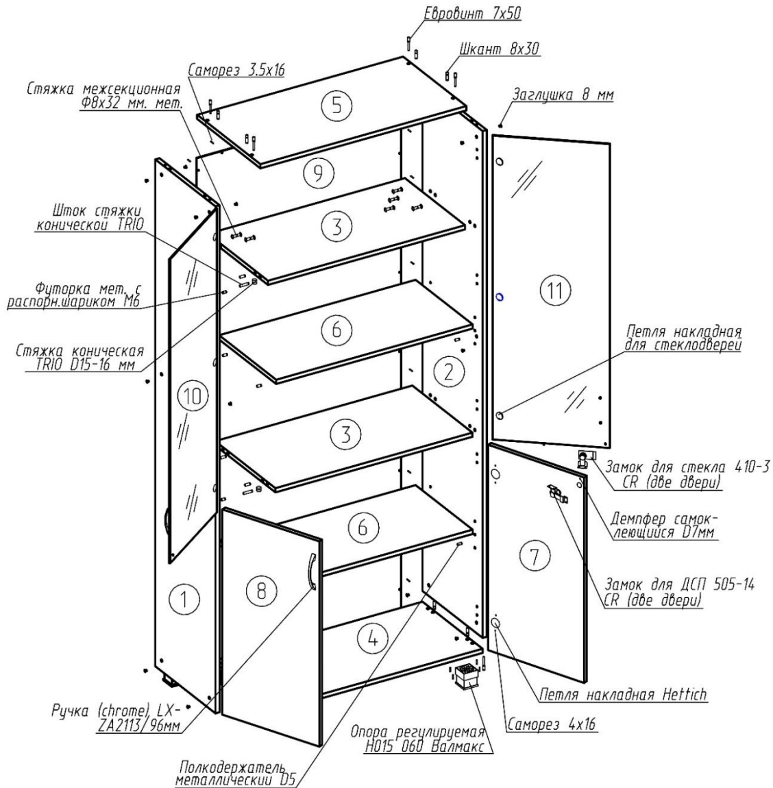
Рисунок 1 – Сборка каркаса
