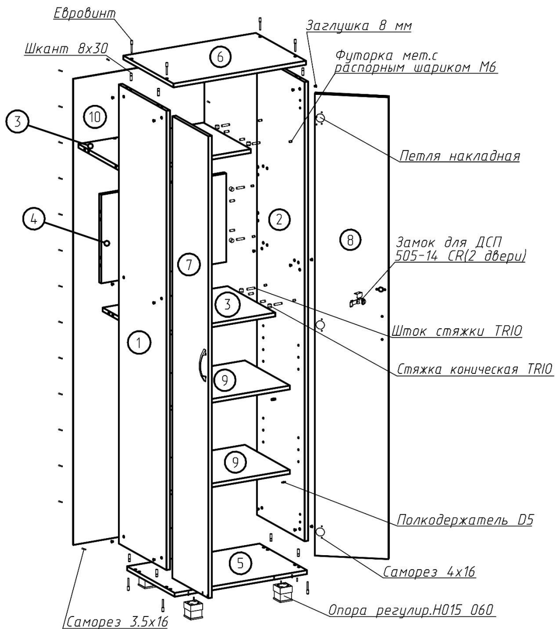
Рисунок 1 – Сборка каркаса
