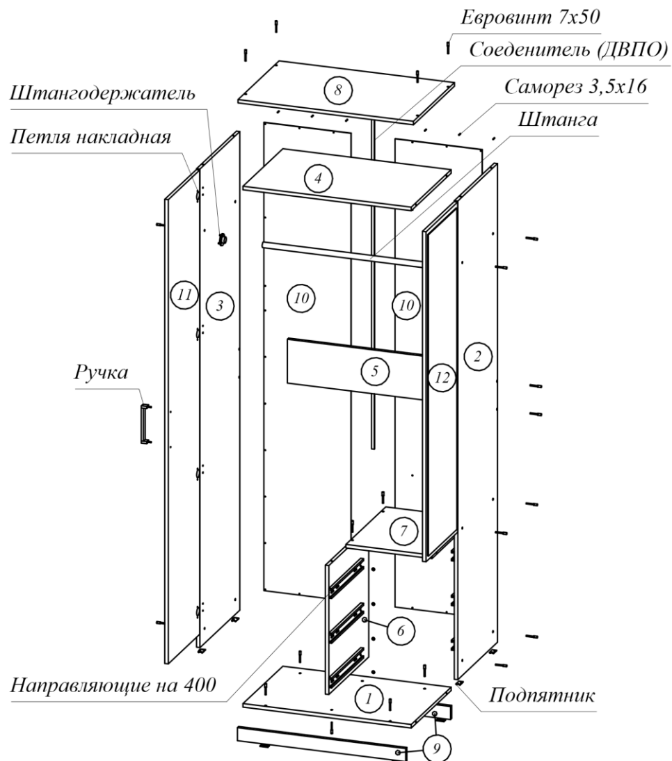
Рисунок 1 – Сборка каркаса
