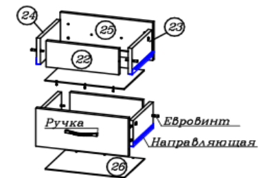
Рисунок 2 – Сборка ящика
