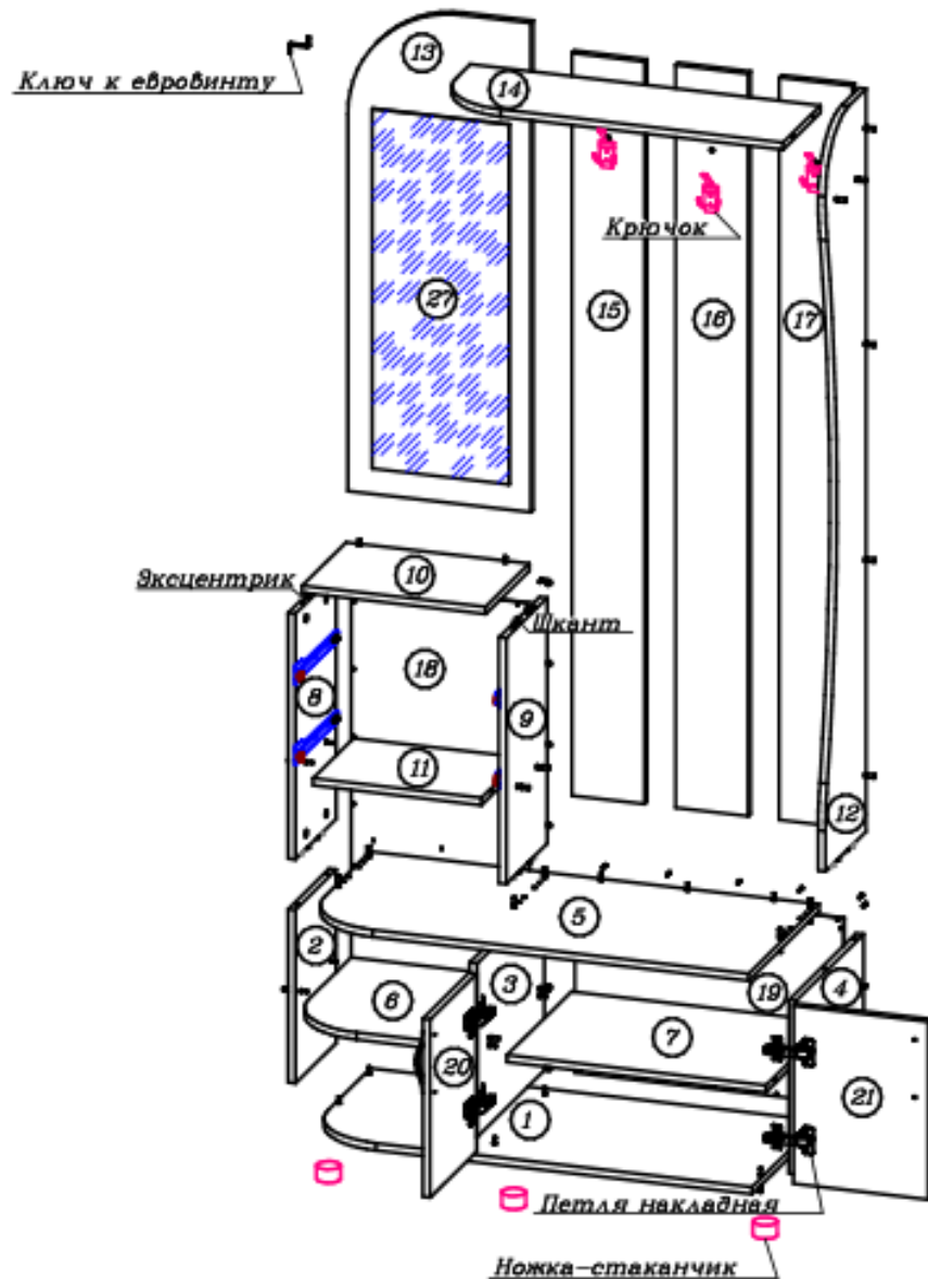
Рисунок 1 – Сборка каркаса
