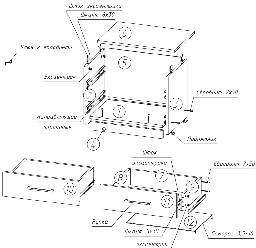
Рисунок 1 – Сборка
