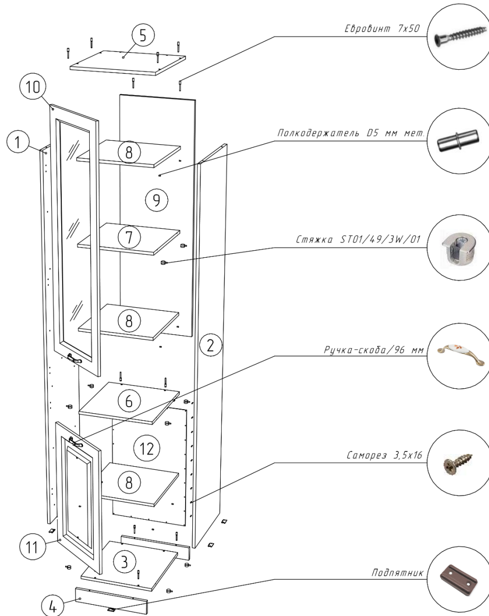
Рисунок 1 – Сборка каркаса
