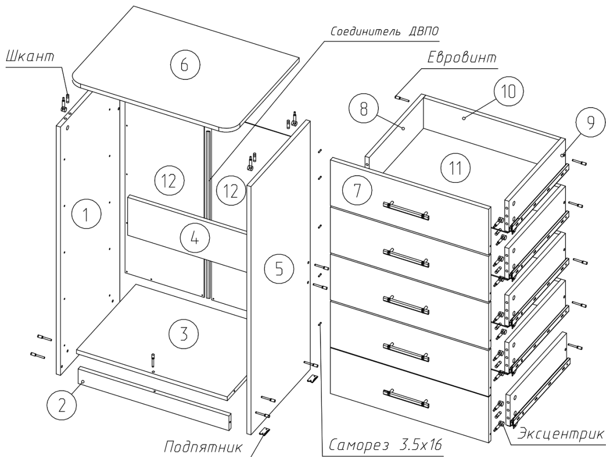
Рисунок 1 – Сборка каркаса и ящиков
