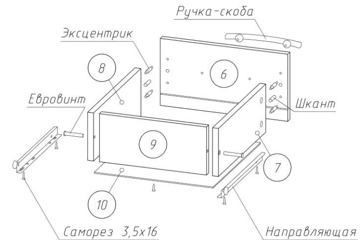
Рисунок 2 – Сборка ящика
