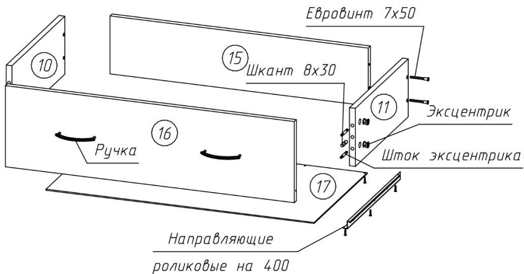
Рисунок 2 – Сборка большого ящика
