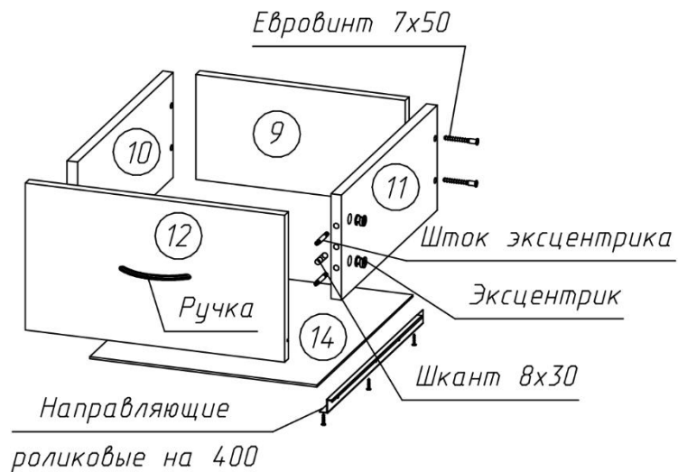
Рисунок 2 – Сборка большого ящика
