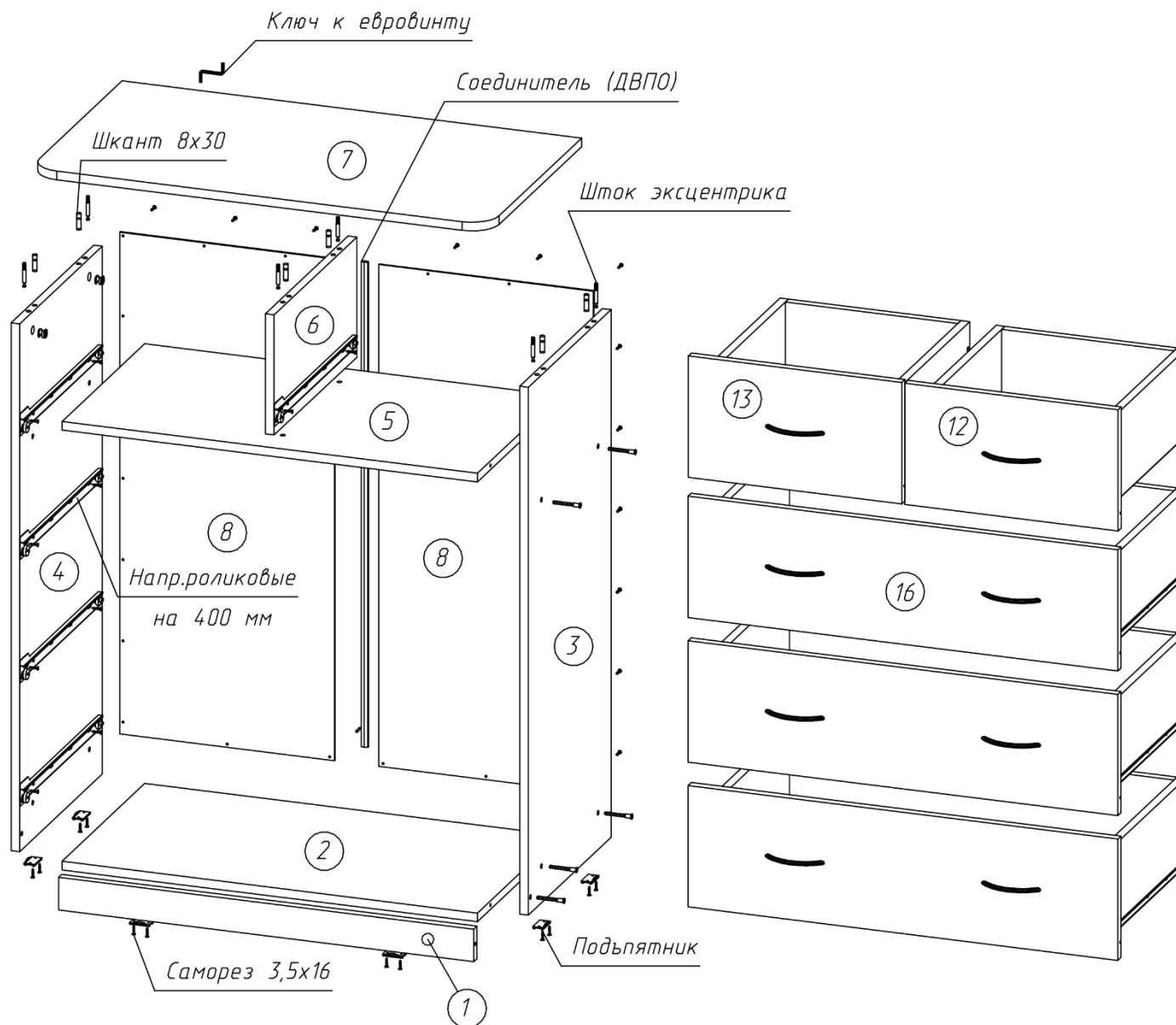
Рисунок 1 – Сборка каркаса
