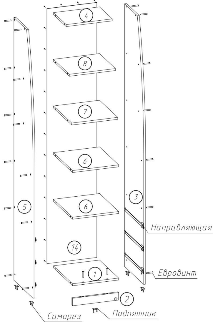
Рисунок 1 – Сборка каркаса
