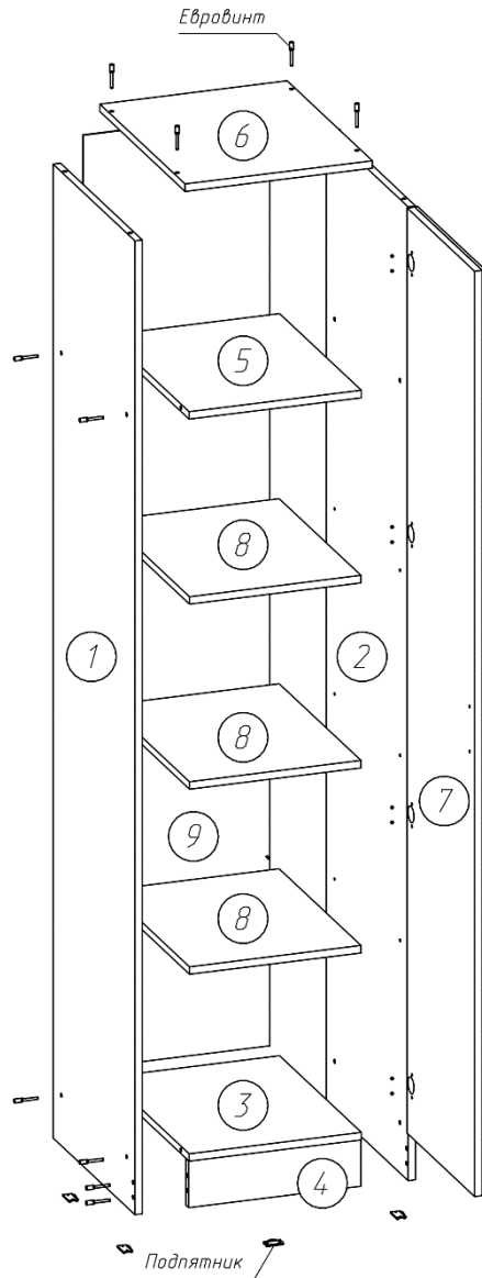
Рисунок 1 – Сборка каркаса
