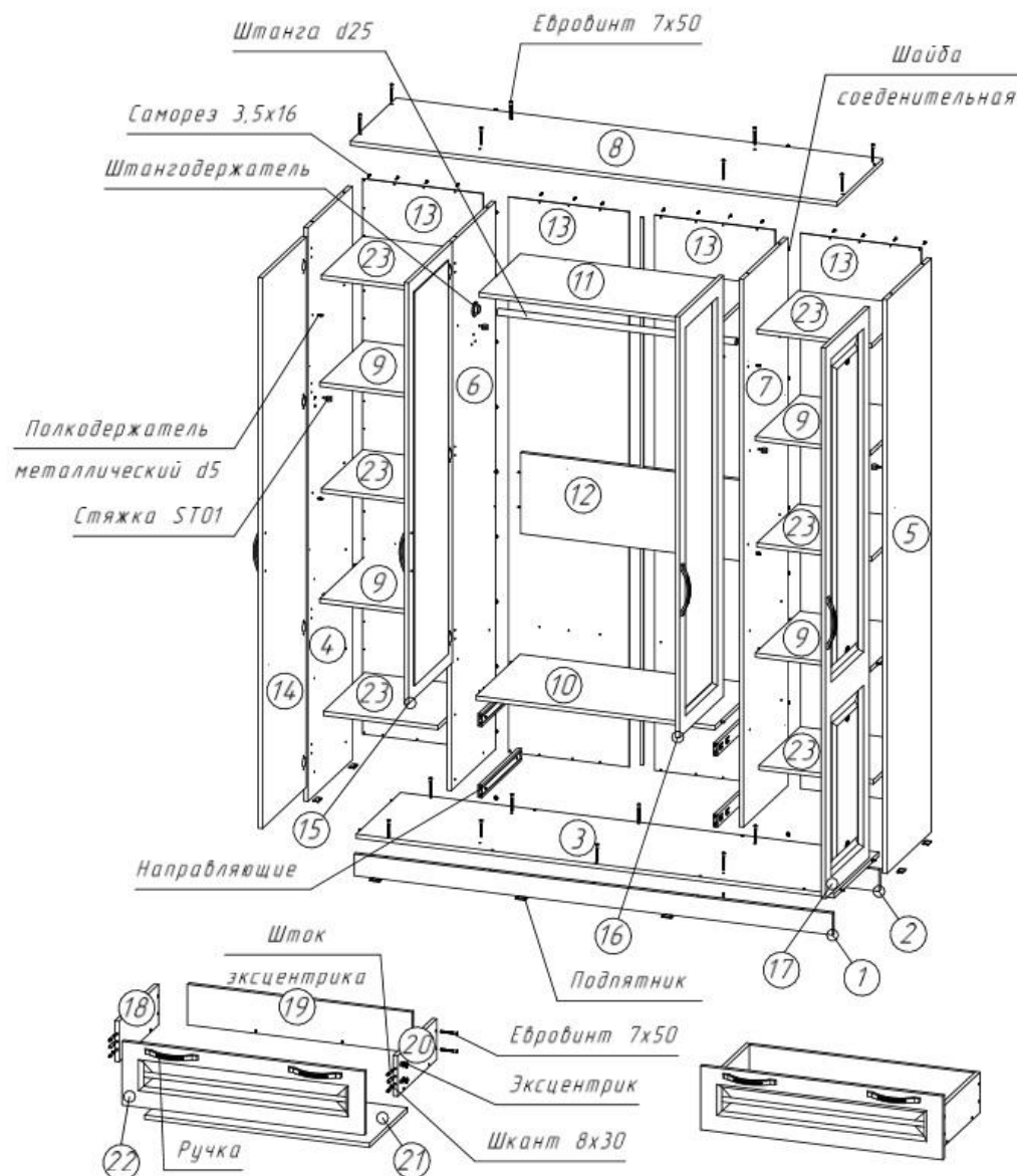
Рисунок 1 – Сборка каркаса
