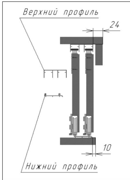
Рисунок 2 – Монтаж профилей и дверей купе, мм
