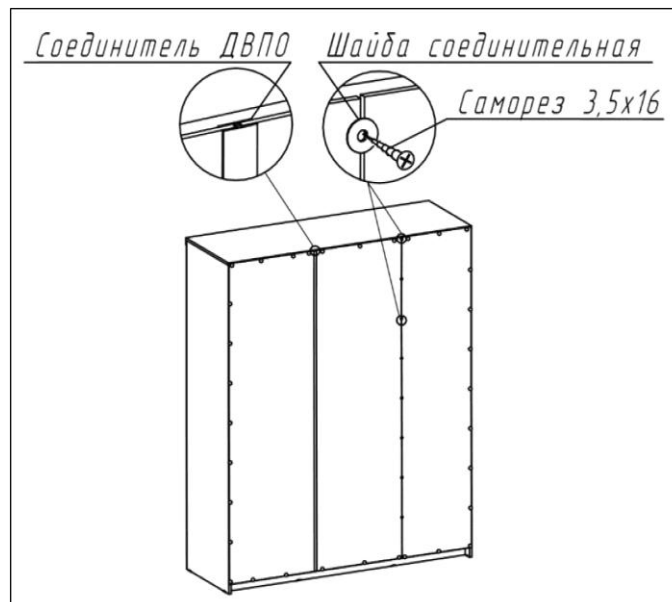
Рисунок 3 – Монтаж ДВПО
