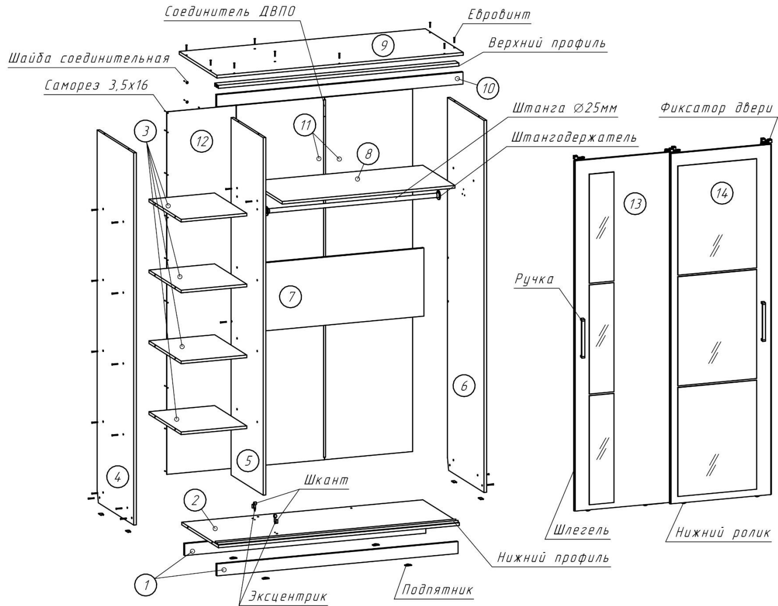
Рисунок 1 – Сборка каркаса
