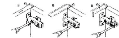
Схема крепления стяжки эксцентриковой усиленной
