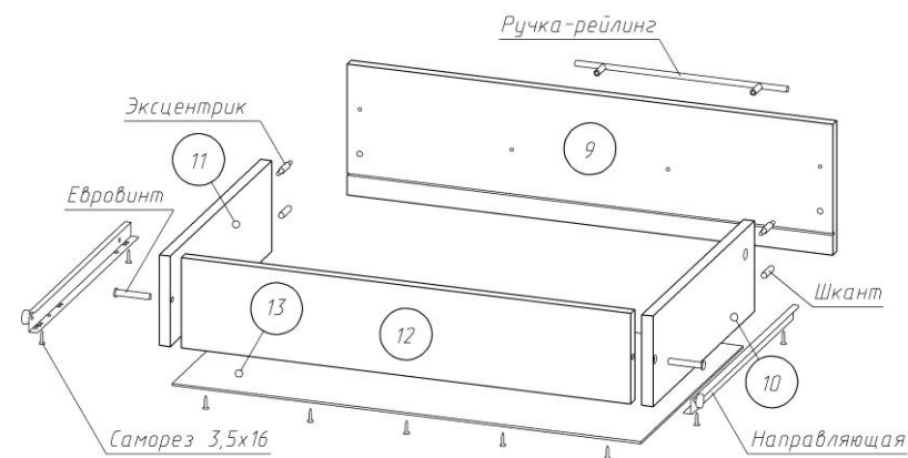
Рисунок 2 – Сборка ящика
