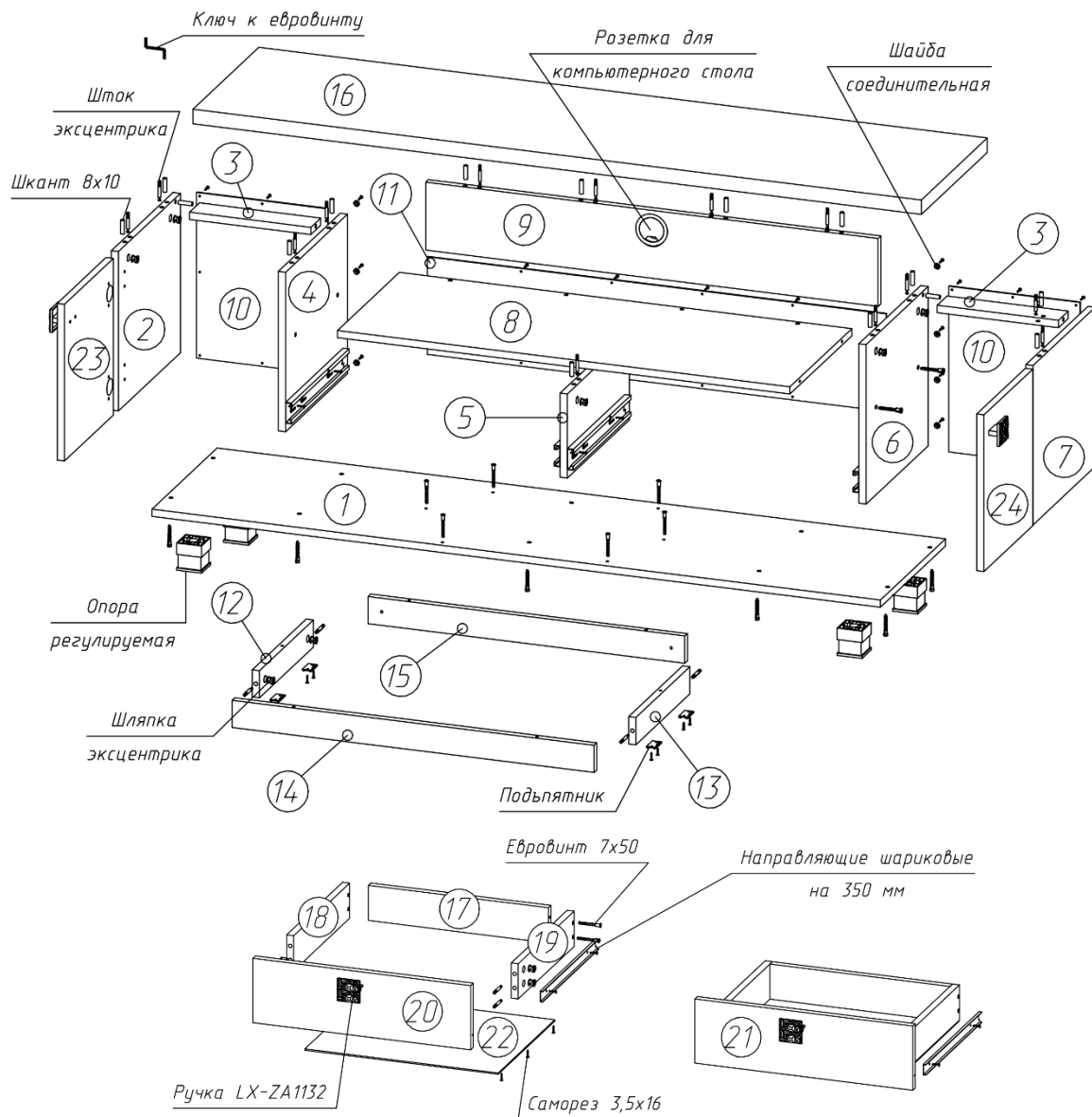
Рисунок 1 – Сборка каркаса и ящика
