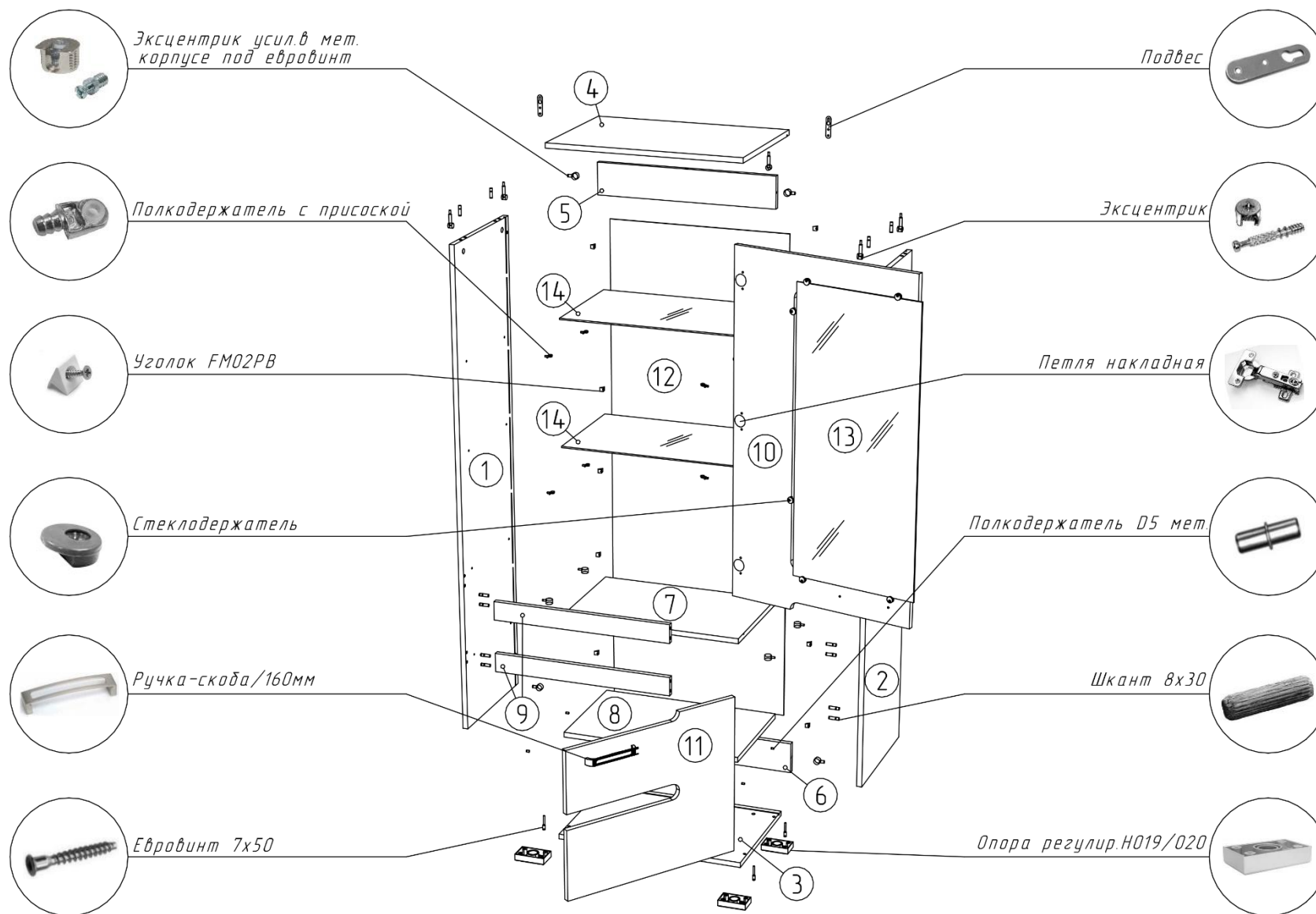
Рисунок 1 – Сборка каркаса
