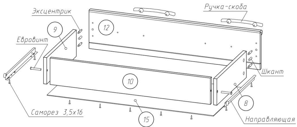
Рисунок 2 – Сборка большого ящика
