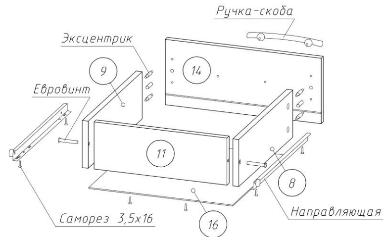
Рисунок 3 – Сборка правого ящика
