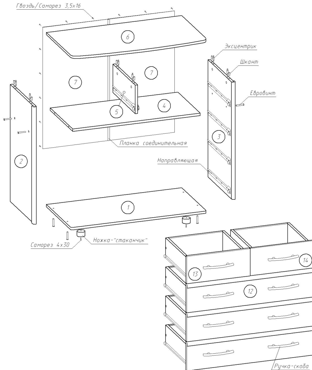
Рисунок 1 – Сборка каркаса
