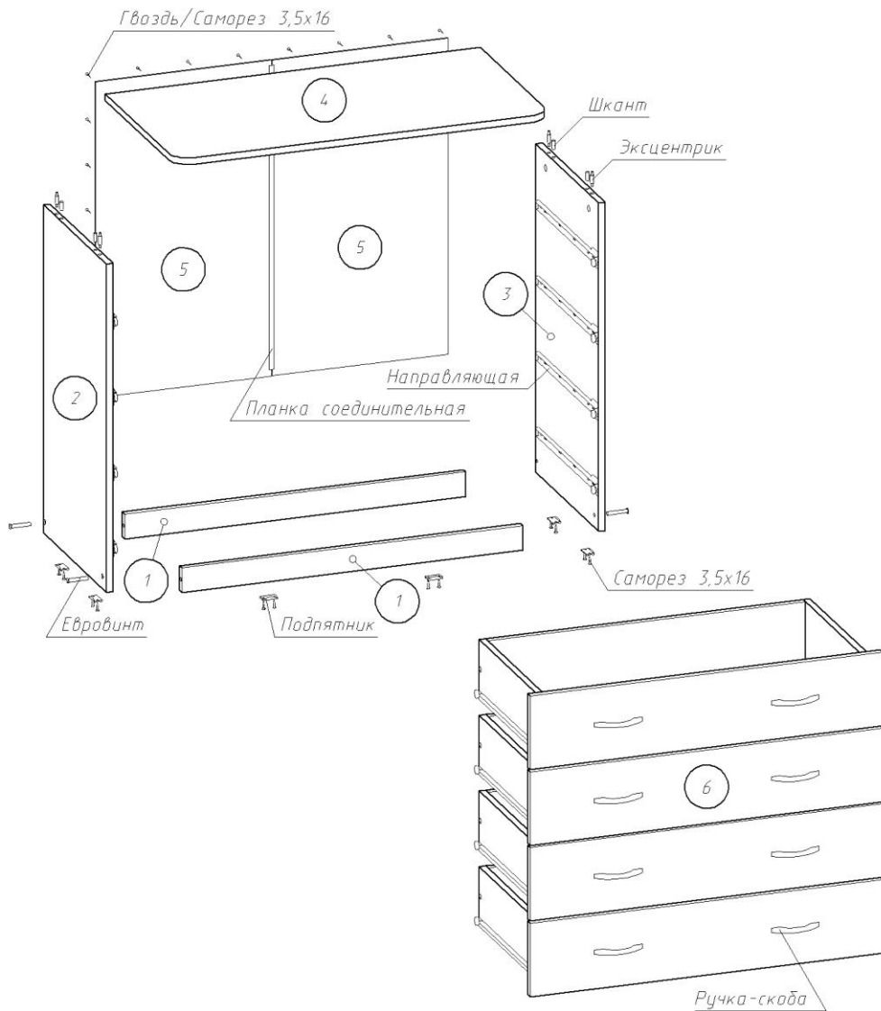
Рисунок 1 – Сборка каркаса
