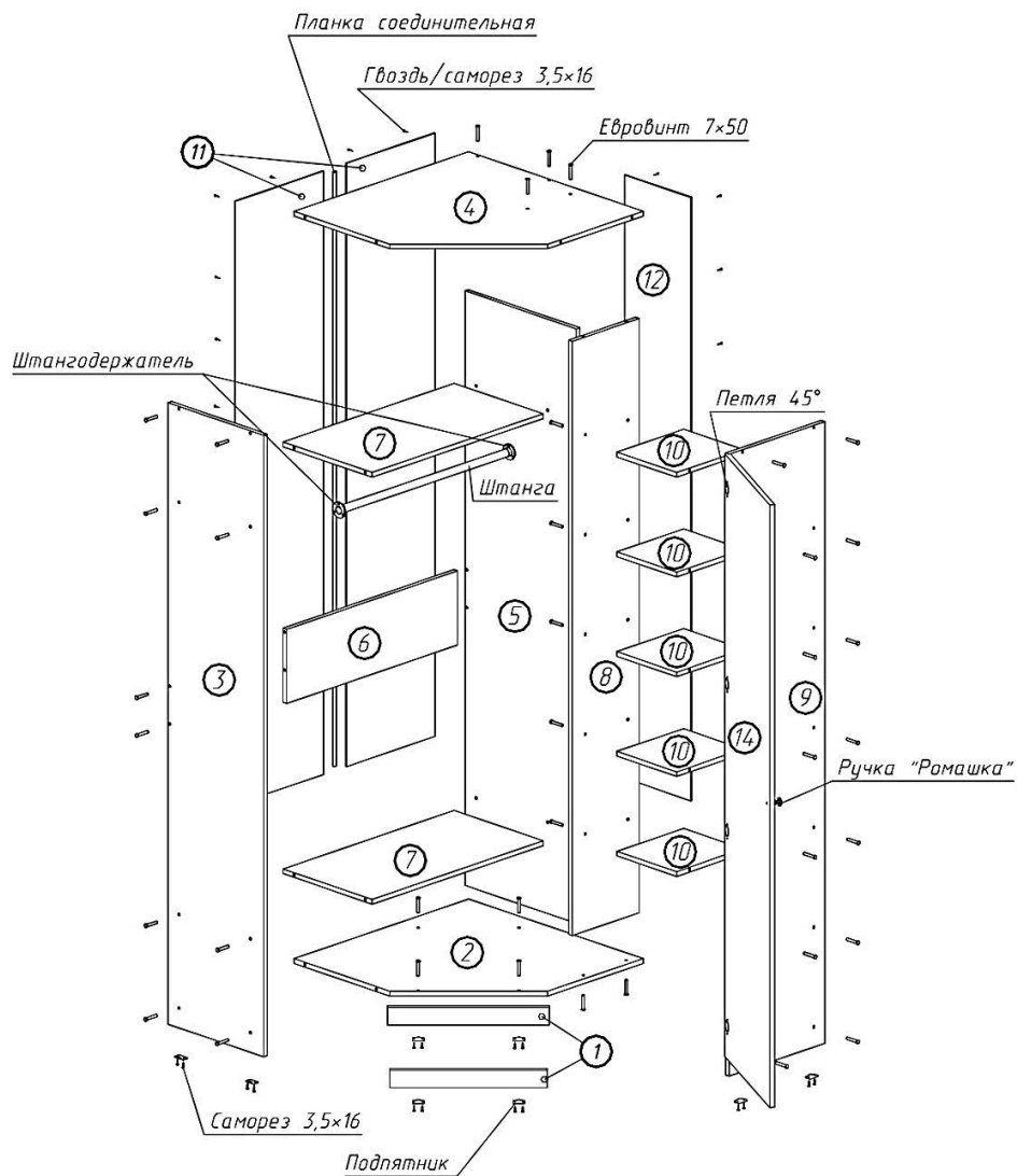
Рисунок 1 – Сборка каркаса
