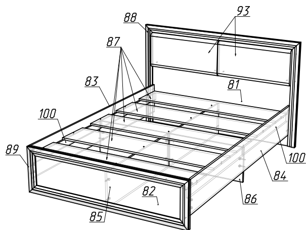
Рис.1 Схема сборки
