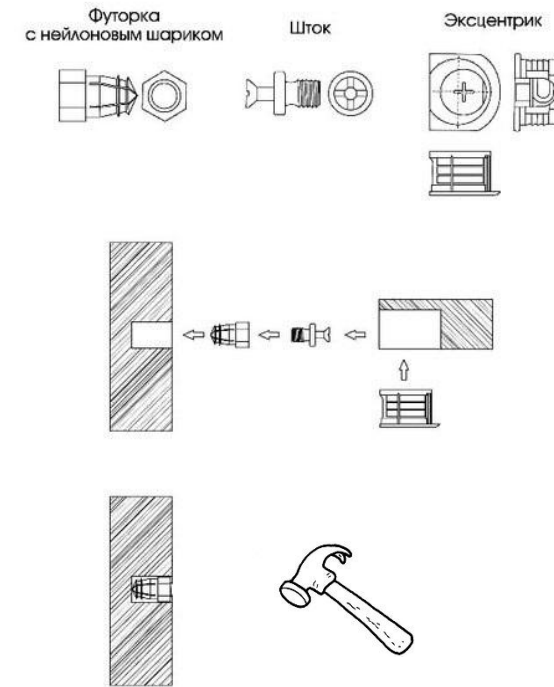
Рисунок 2 – Монтаж футорки
