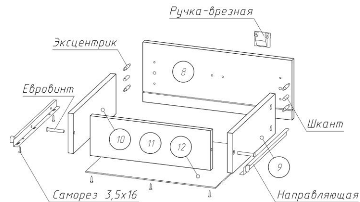
Рисунок 2 – Сборка ящика
