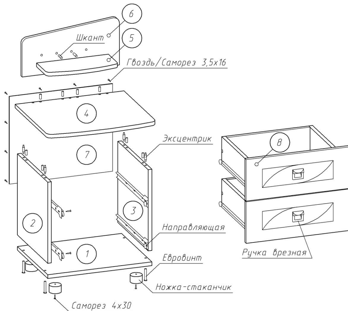
Рисунок 1 – Сборка каркаса
