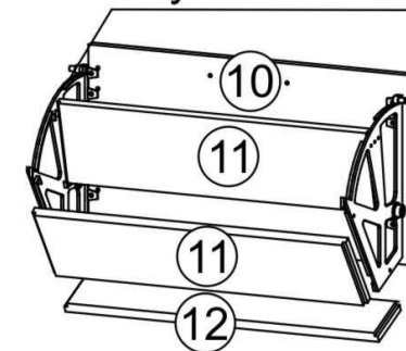
Рисунок 2 – Сборка обувницы
