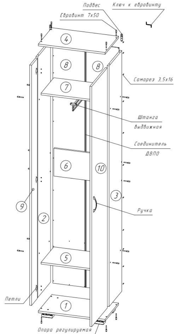
Рисунок 1 – Сборка шкафа
