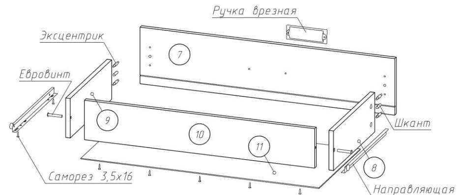
Рисунок 2 – Сборка ящика
