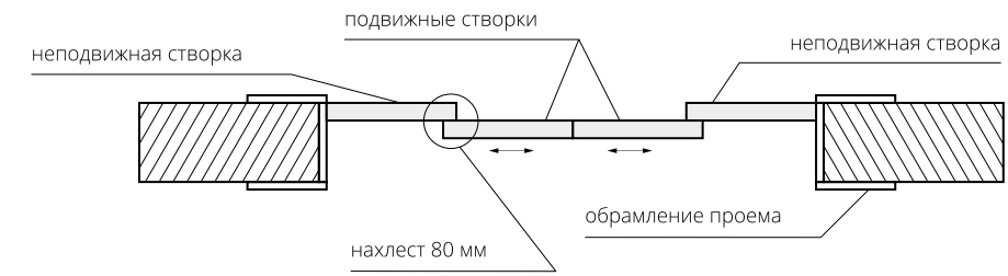
Установка перегородки в проем
