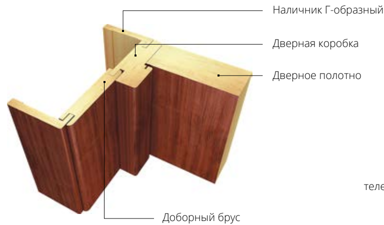
Дверной угол
