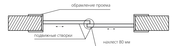
Установка перегородки в проем
