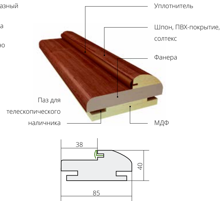
Короб плоский (тип 1)
