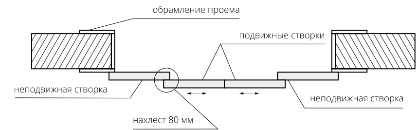
Установка перегородки вне проема
