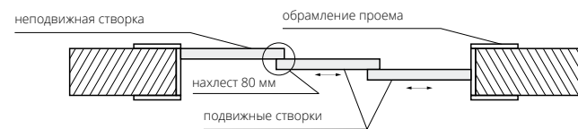
Установка перегородки в проем
