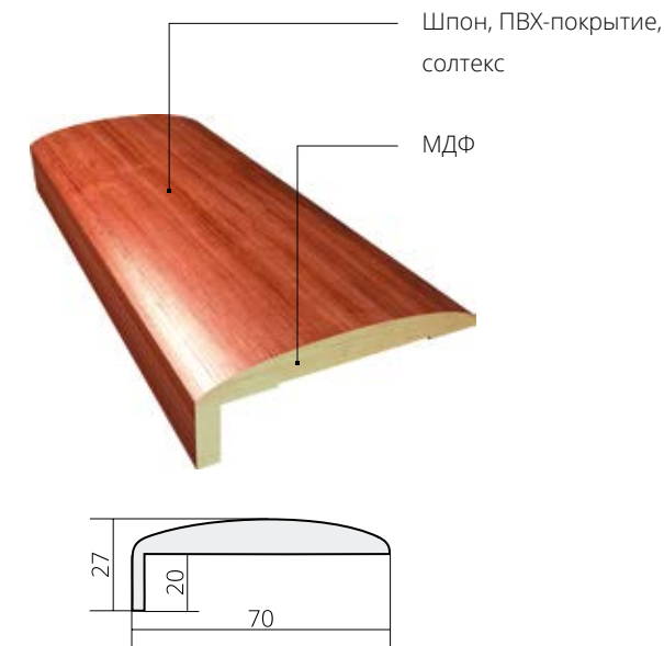
Наличник полукруглый (тип 2)
