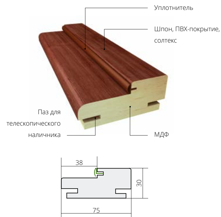
Короб плоский (тип 1)
