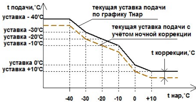
рис. 5 Задание подачи отопления и ночная коррекция
