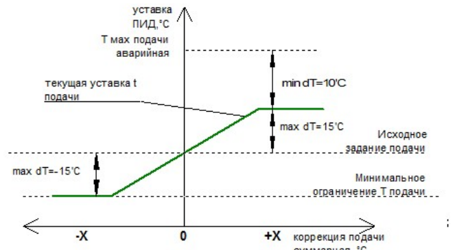
Рис. 8. Ограничение уставки общее, без учёта ночной коррекции.
