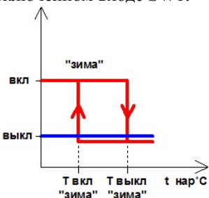
Рис. 9. Переключение режимов «зима»-«лето».
