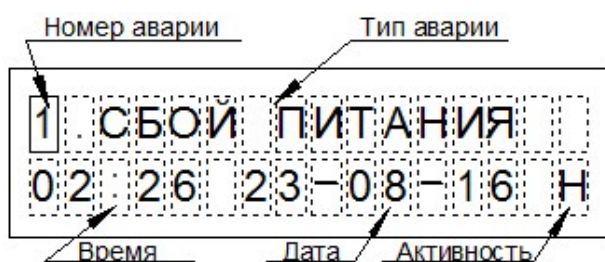
Рис. 11 Меню журнала аварий установки.
