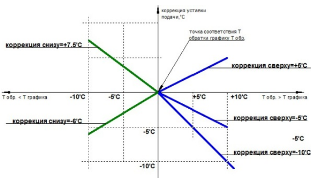
Рис. 7 Расчёт коррекции по обратной воде.
