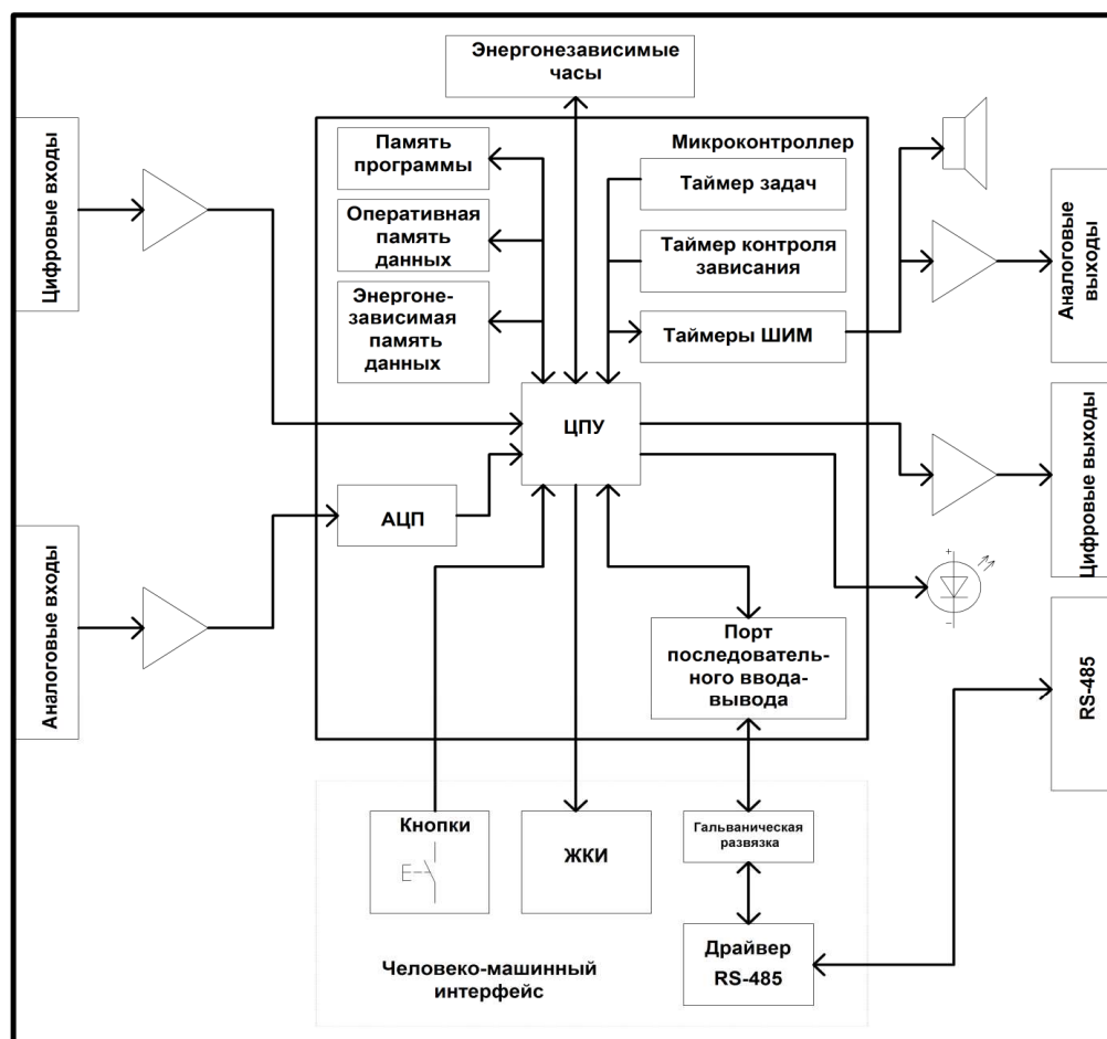
рис.3. Аппаратная модель контроллера.
