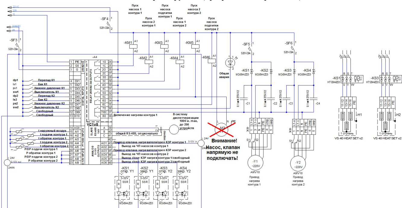
Рис.1 Схема внешних подключений к контроллеру VC1 (программная версия HC1).
