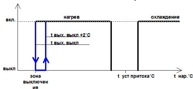
Рис. 6а Температурный график работы роторного рекуператора.
