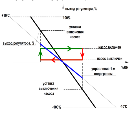
Рис. 7 График работы форсуночного увлажнителя.
