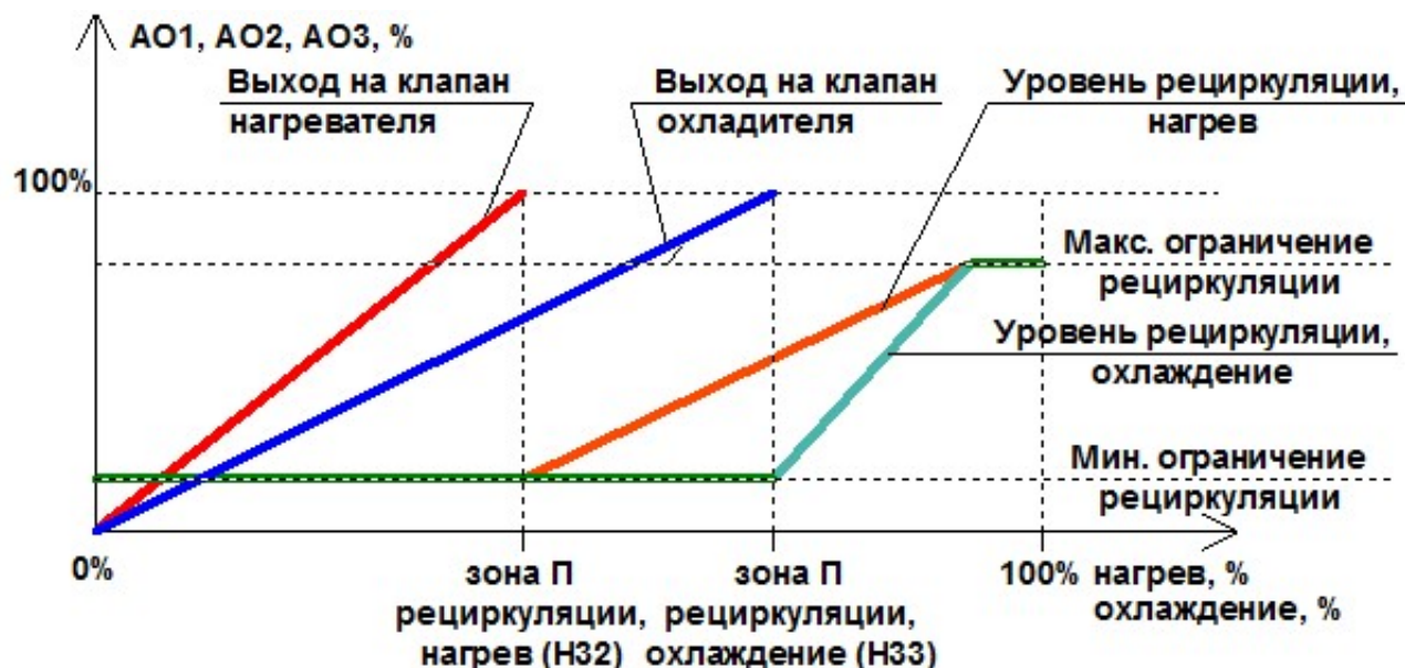
Рис. 7б. Работа рециркуляции в прямом режиме.
