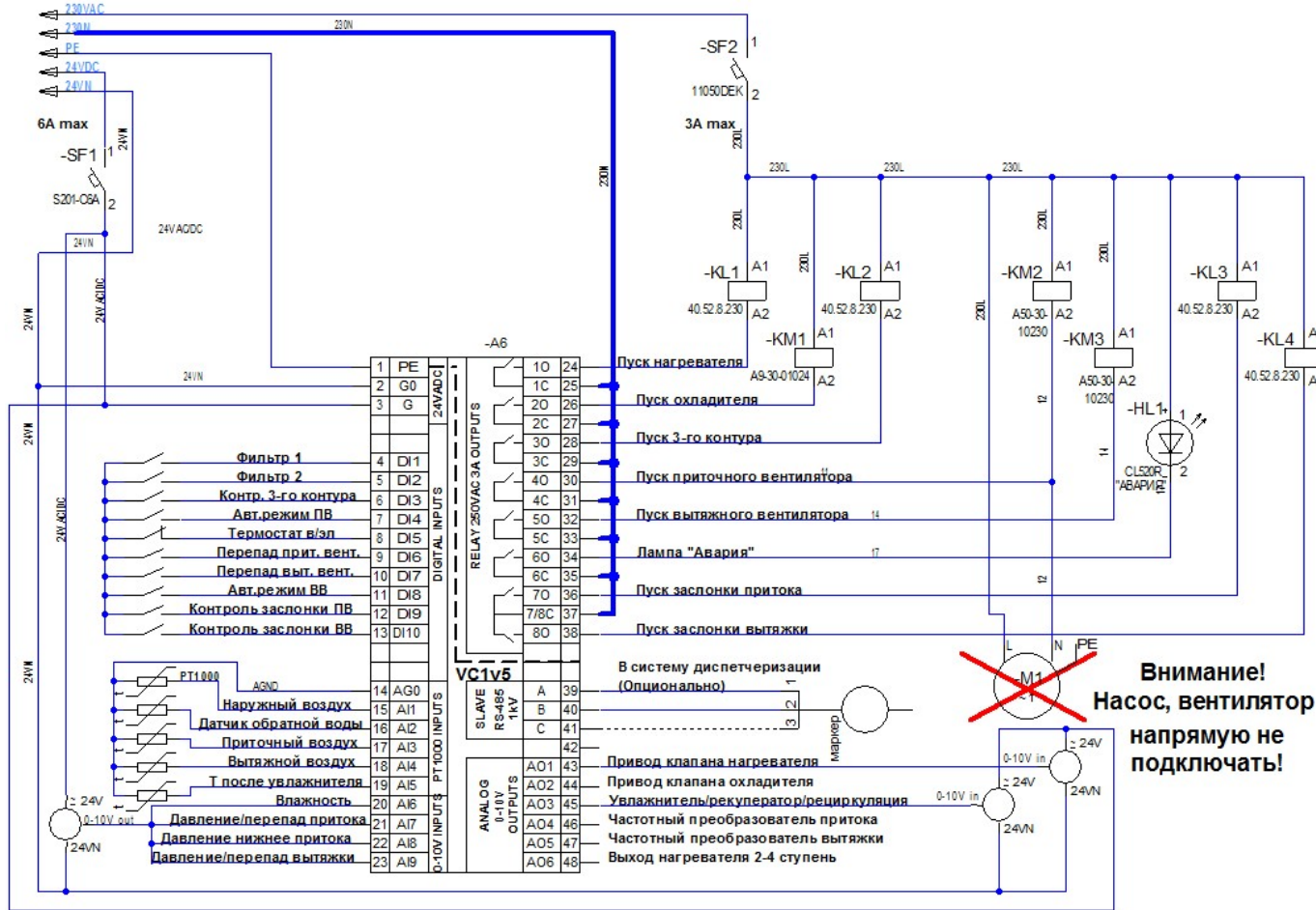
Рис.1а Схема внешних подключений к контроллеру VC1.
