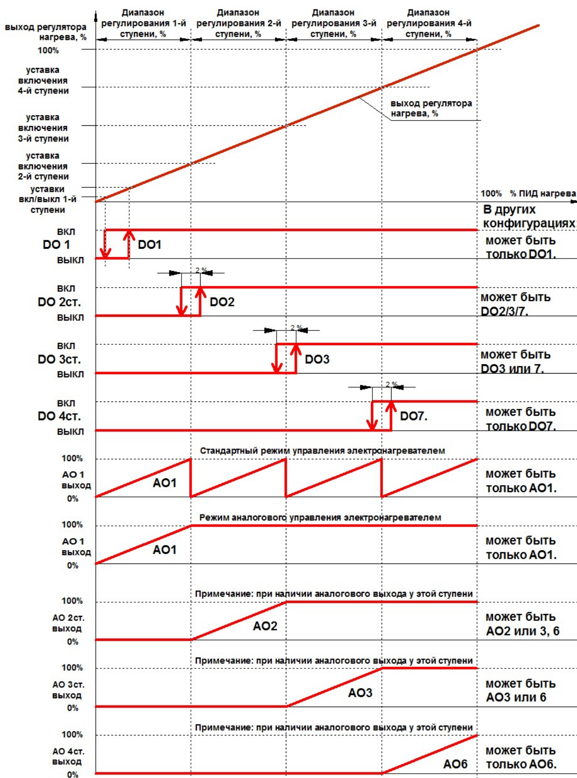
рис. 2. Логика работы 4-ступенчатого электронагревателя.
