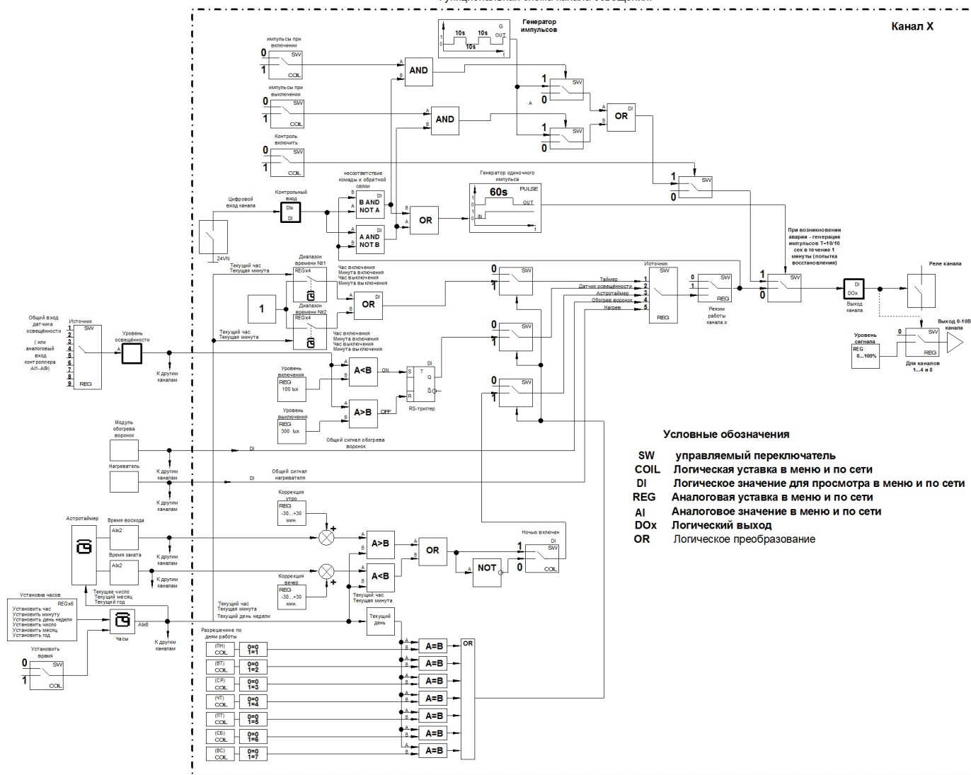
Рис. 5. Структурная схема канала освещения.
