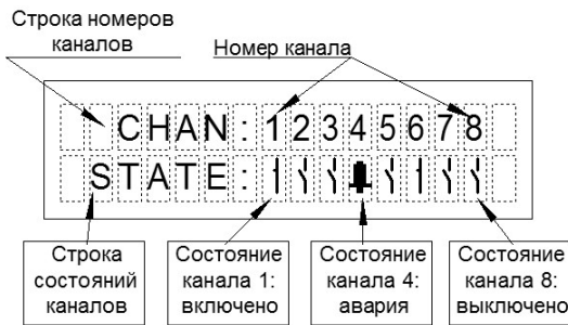
рис. 9. Главное меню.
