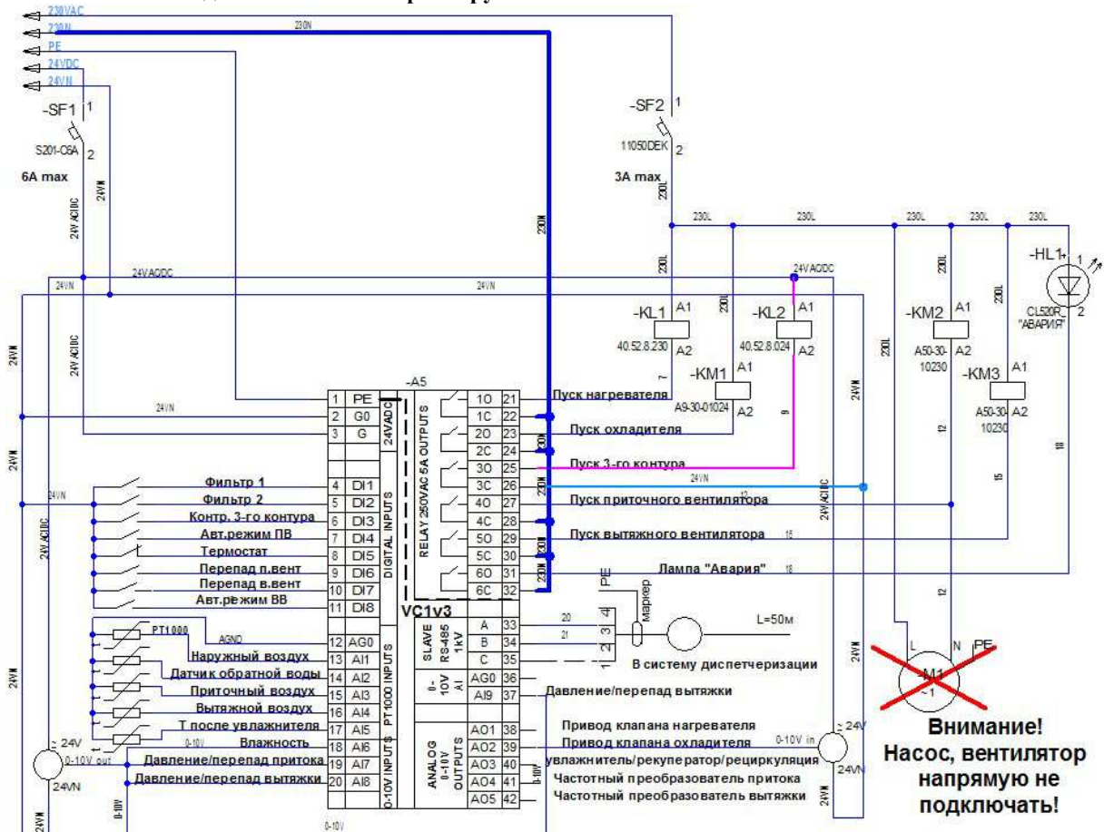
Рис.1 Схема внешних подключений к контроллеру VC1.
