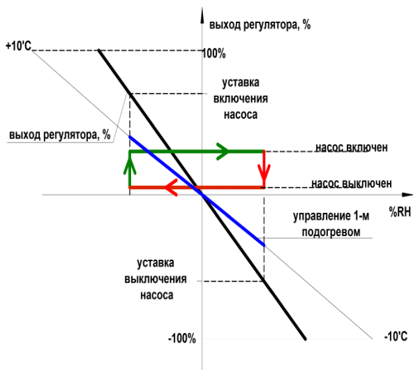
Рис. 7 График работы форсуночного увлажнителя.
