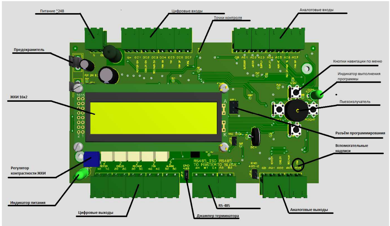
Рис 2. Внешний вид контроллера со снятой крышкой.
