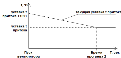
Рис. 4 График работы прогрева при пуске.
