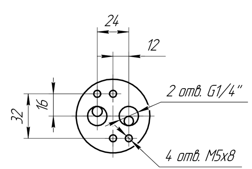
Посадочная площадка G1/4" NAMUR
