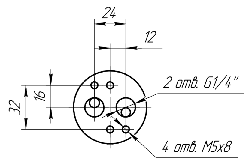
Посадочная площадка G1/4" NAMUR
