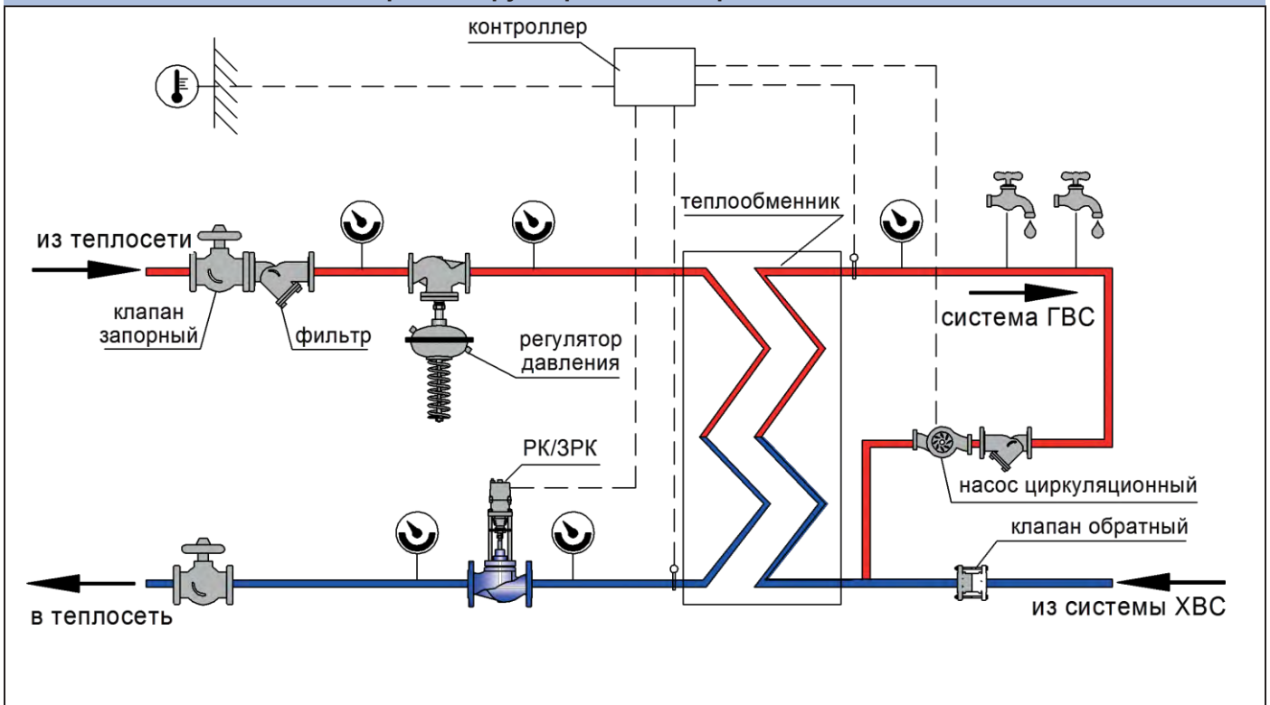
На обратном трубопроводе в закрытой системе ГВС
