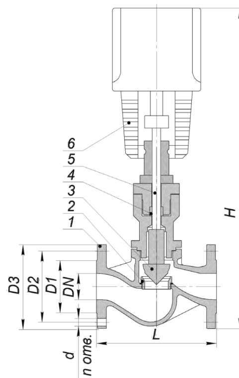
Клапан на пар с приводом ТНК
