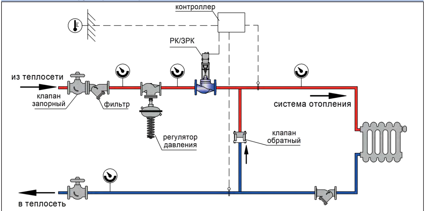
На подающем трубопроводе при зависимом присоединении системы отопления к тепловой сети
