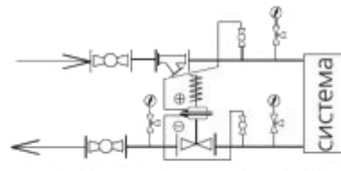
Установка регулятора перепада давления на обратном трубопроводе
