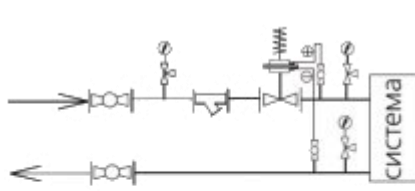
Установка регулятора перепада давления на подающем трубопроводе
