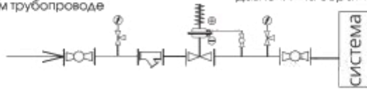
Установка регулятора давления "после себя" на подающем трубопроводе
