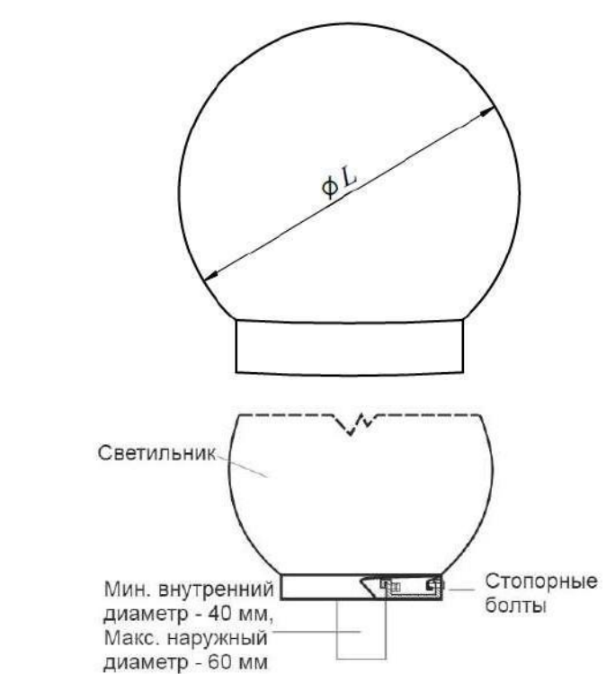
Консольный для шаров Применяется для светильников серии «Шар»
