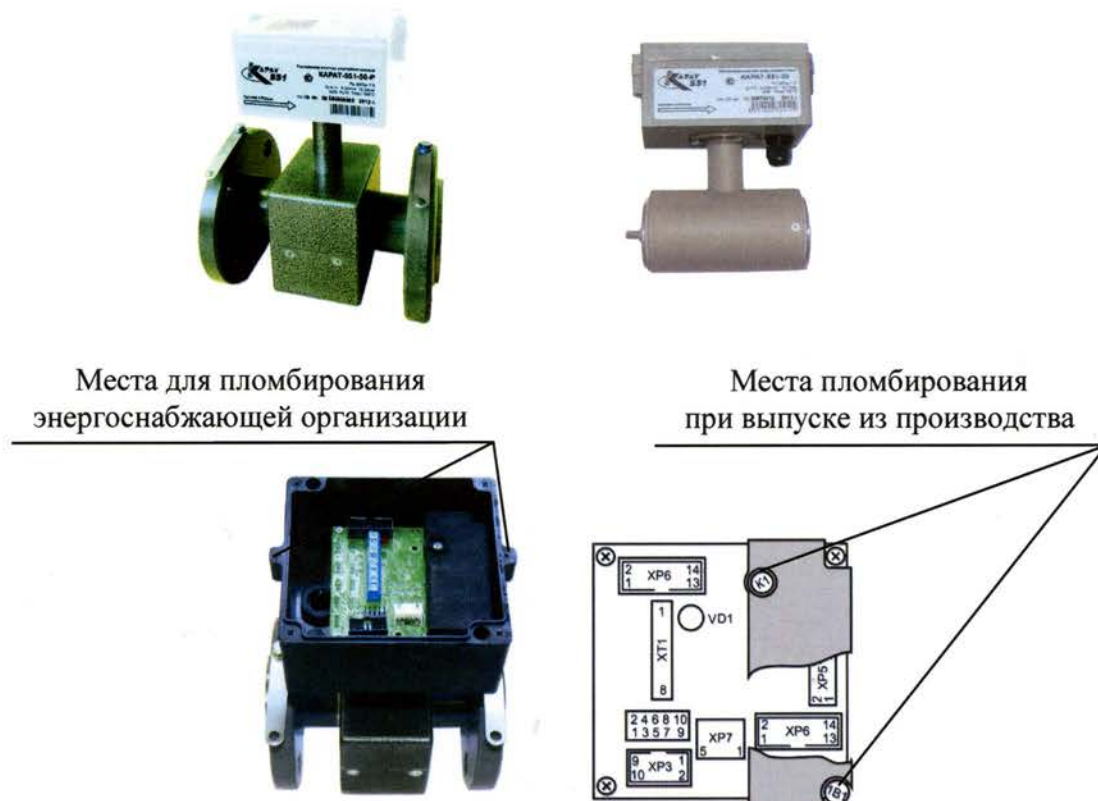
Рисунок 1 – Внешний вид расходомеров КАРАТ- 551 и места их пломбирования
