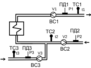
Рисунок В.6 – Схема на источнике
