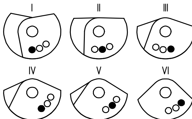
Рисунок 4. Схема регулировки статического момента ступенчато регулируемых дебалансов вибраторов ИВ-20-50, ИВ-20-50Н, ИВ-107Н.
