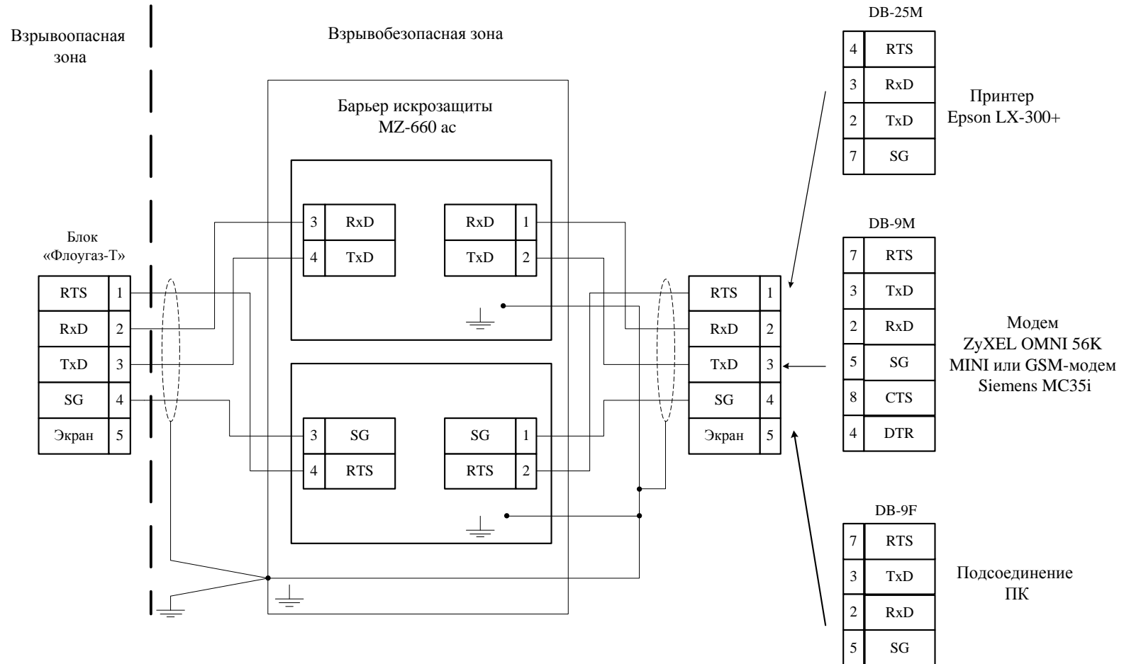
Рисунок Б 4 Схема подключения блока к внешним устройствам (ПК, модем, принтер) во взрывоопасной зоне
